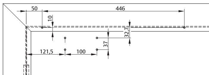
Schéma de fixation pour pose sur la porte côté opposé aux paumelles
