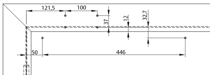
Schéma de fixation pour pose sur l'huissierie côté opposé aux paumelles
