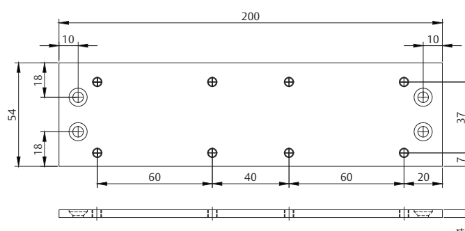
Plaque de montage A280
