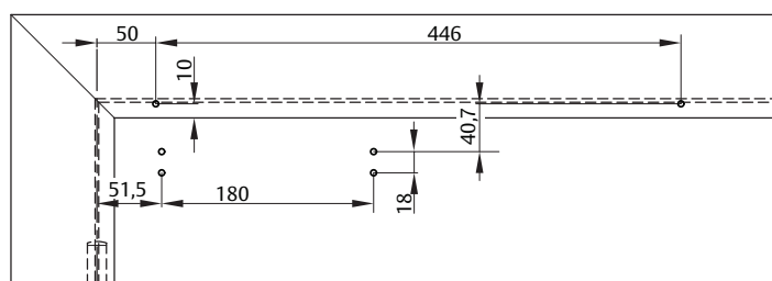
Schéma de fixation sur la porte côté opposé aux paumelles avec plaque de montage
