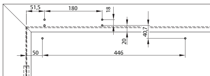
Schéma de fixation sur l'huissierie côté opposé aux paumelles avec plaque de montage
